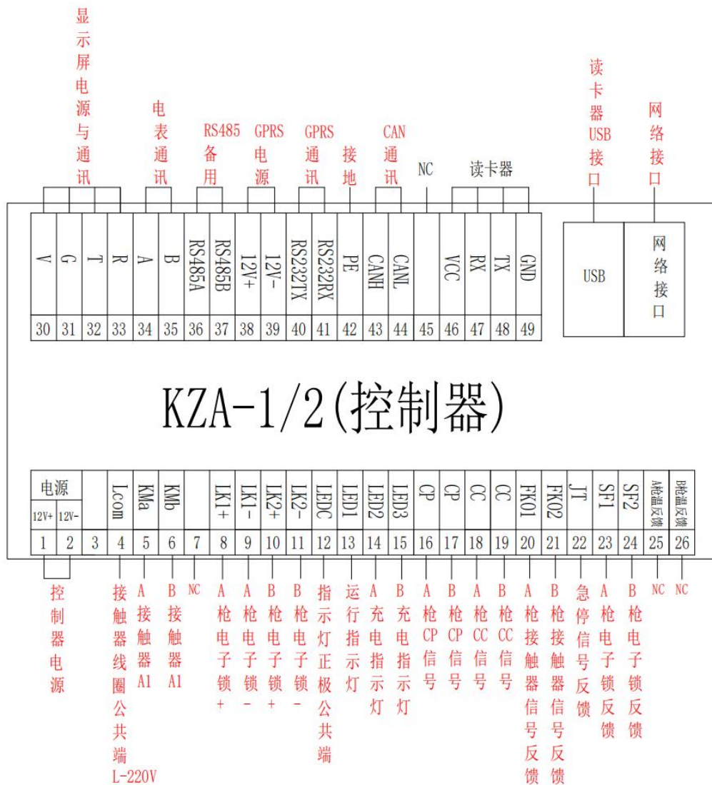
QGDZA-1/2 接口示意图
